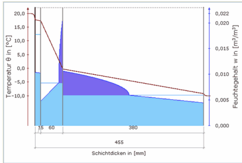
Abbildung 7: Mit dem COND-Verfahren berechnete Feuchteverteilung am Ende der Kondensationsperiode
