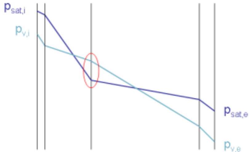
Abbildung 4: Sättigungsdampfdruck- und Dampfdruckprofile mit Kondensationsebene
