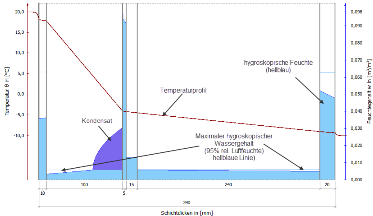
Abbildung 14: COND Diagramm mit Feuchtfeld
