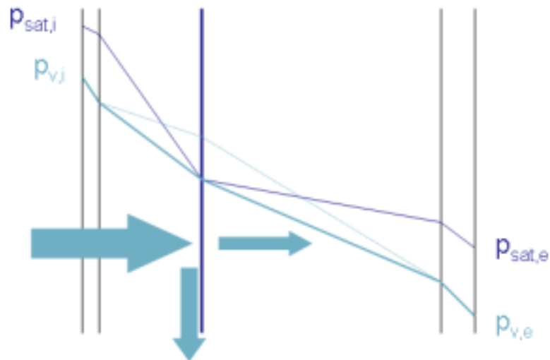
Abbildung 5: Aus dem Ungleichgewicht der Dampfströme zur und von der Kondensatebene weg wird Kondensat berechnet (Glaser)
