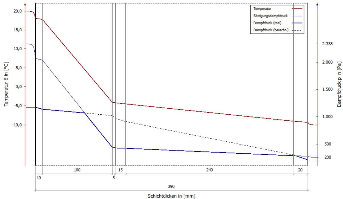
Abbildung 15: COND Diagram mit Dampfdrücken
