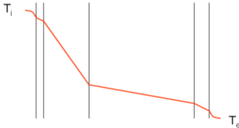
Abbildung 3: Stationäres Temperaturprofil in der Kondensationsperiode
