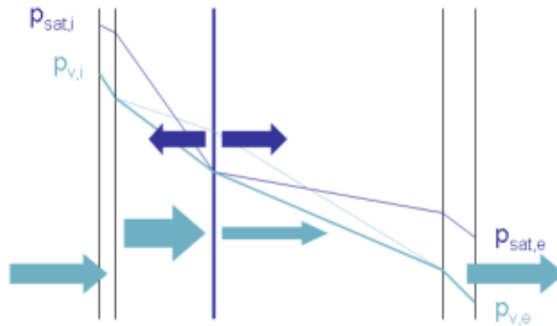
Abbildung 6: Dampfströme (hellblau) und von der Kondensatebene wegführende Flüssigwasserströme (dunkelblau), im stationären Zustand sind Dampfströme in die Konstruktion und aus der Konstruktion heraus gleich groß
